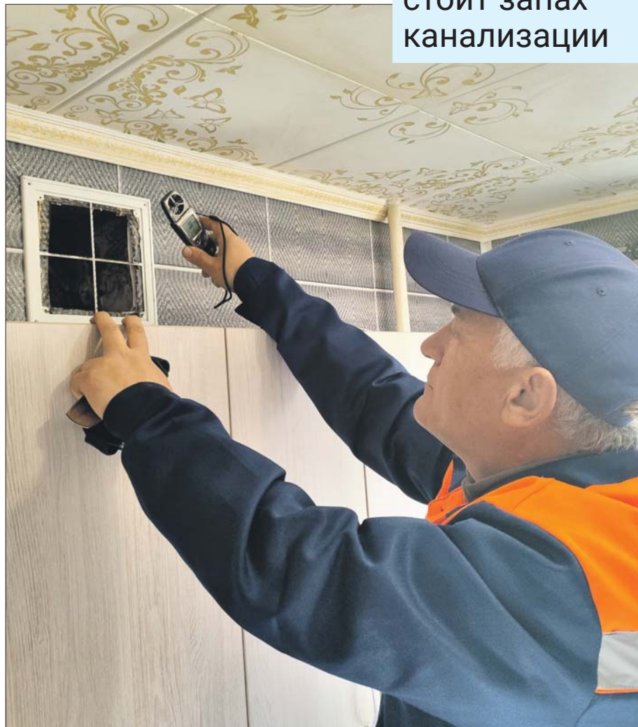
Мастер измеряет скорость движения воздуха ручным анемометром — показатели в норме
