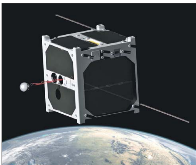
Тормозное устройство разработано для малых космических аппаратов формата CubeSat
